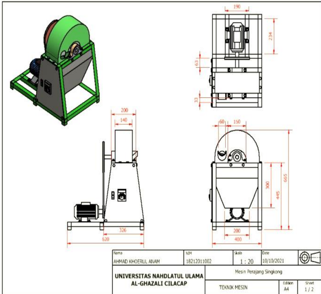
Gambar Teknik Mesin Perajang Singkong
